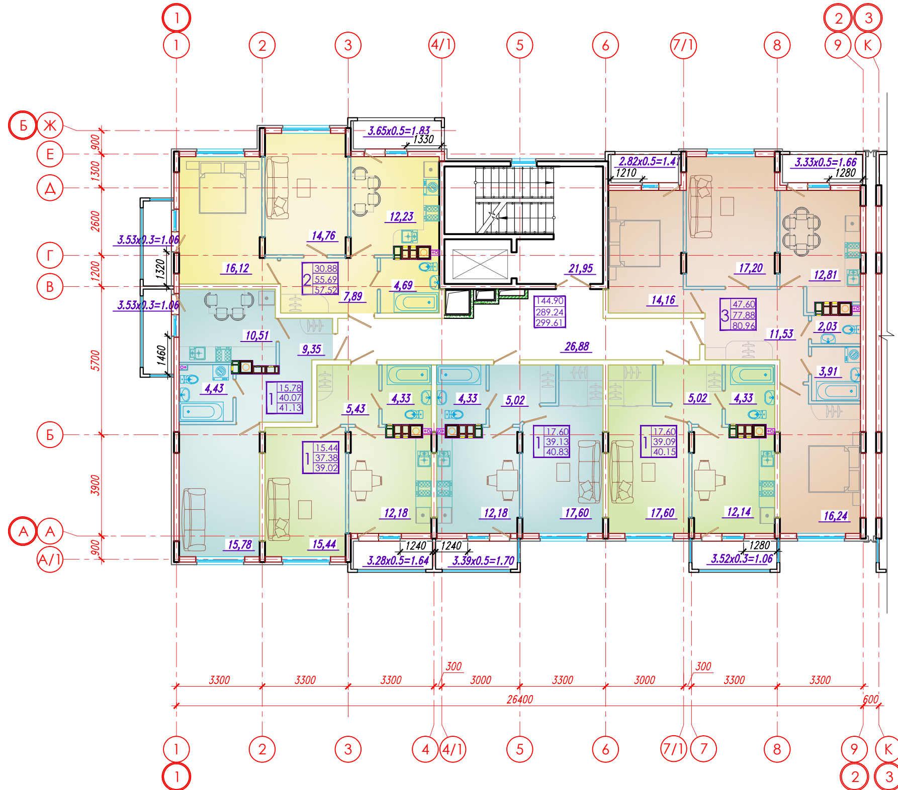
Литер Г, блок-секция 3 План типового этажа
